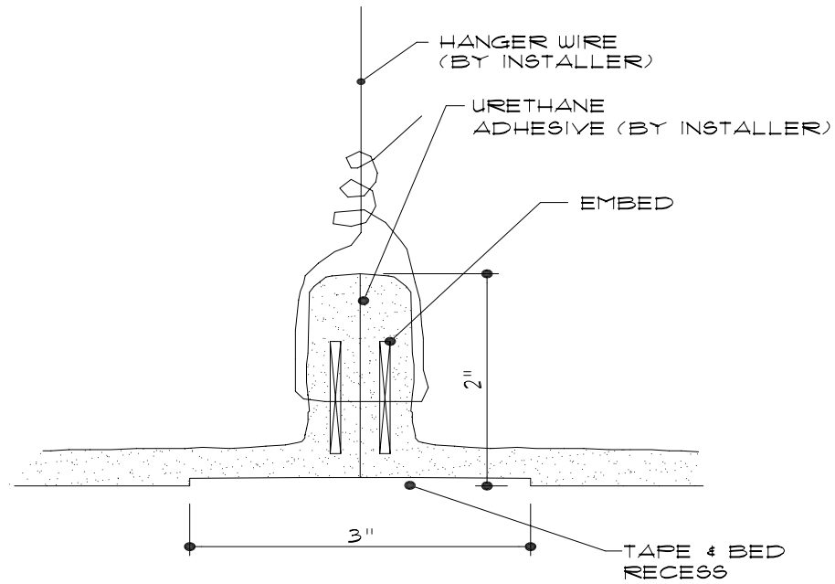
1 6 TYP. TAPE & BED RECESS N.T.S.
