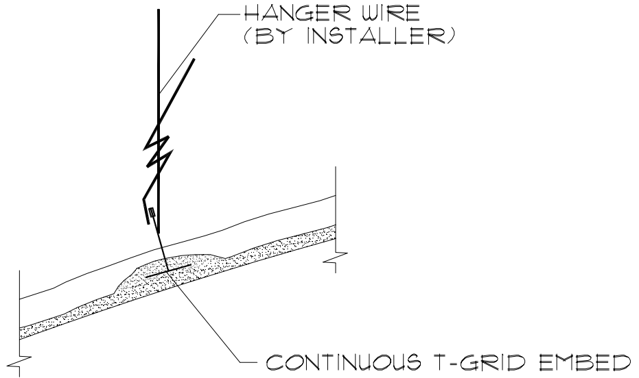
2 6 G.R.G. DOME HANGER / EMBED DETAIL N.T.S.
