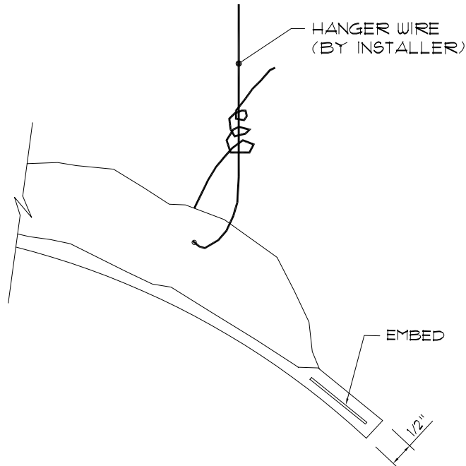
2/2 SECTION @ GRG DOME EDGE N.T.S.
