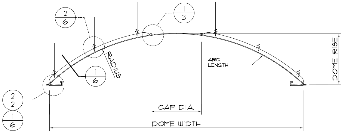
1/2 DOME SECTION N.T.S.
