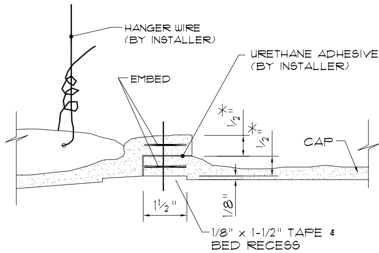
1 SECTION @ GRG DOME CAP 3 N.T.S.
