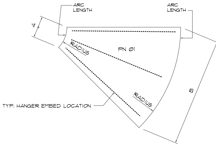
2 GRG DOME GEOMETRY - PN 01 3 N.T.S.
